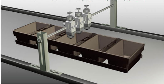
SMX 食品脱模油自动喷涂机
